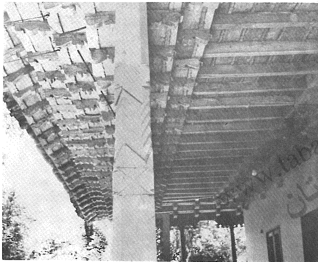
( عکس شماره ۲۱۳ ) چکش گردانها و پشتۀ بام بقعۀ امیر حیدر و امیر احمد در دهکده امیر بنده رانکوه
