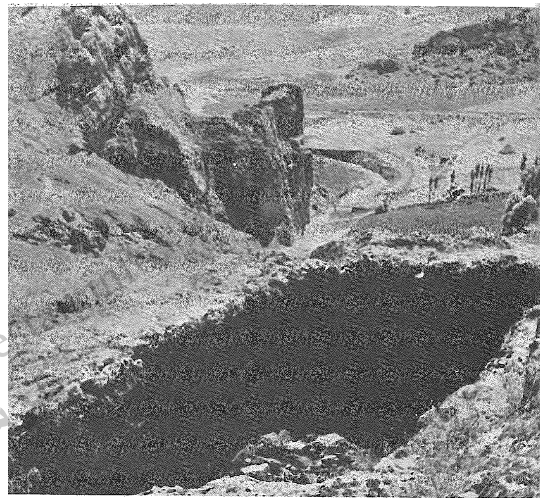
(عکس شماره ۲۴۶) آب انبار شماره سه قلعه گرماور در دهکده گرمسا و سمام
