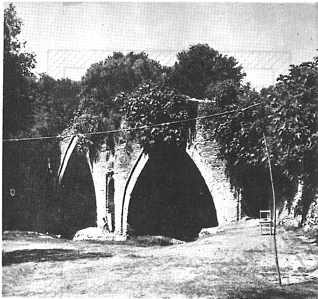
(عکس شماره ۱۲۲) نمای خشت پل بر رودخانه سیم رود نزدیک شهر لاهیجان
