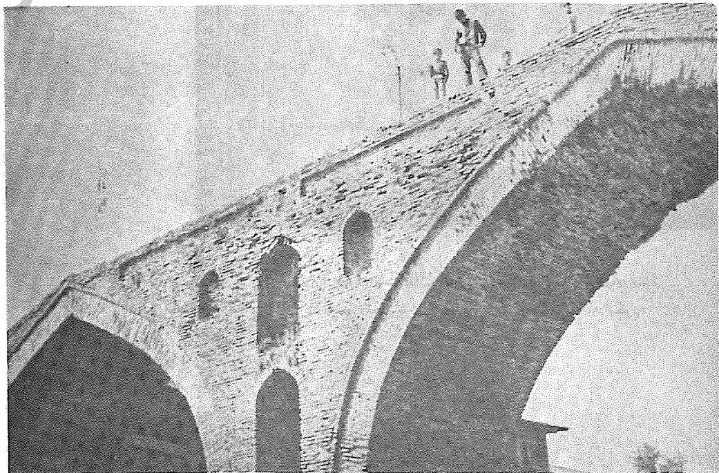
(عکس شماره ۱۸۵) طاقهای جناقی چشمه‌های خشت پل لنگرود برودخانه لنگرود درفشکالی محله لنگرود
